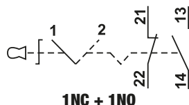
Kétállású rugóvisszatérítéses
