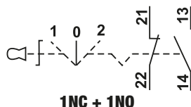
Háromállású rugóvisszatérítéses
