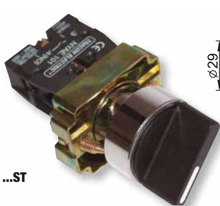
Kétállású normál
