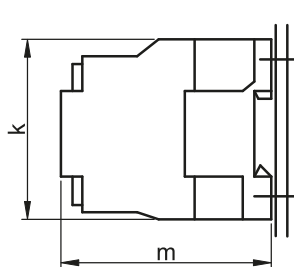
Szerelőlapra szerelve
