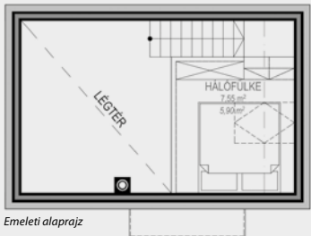
Emelet alaprajz
