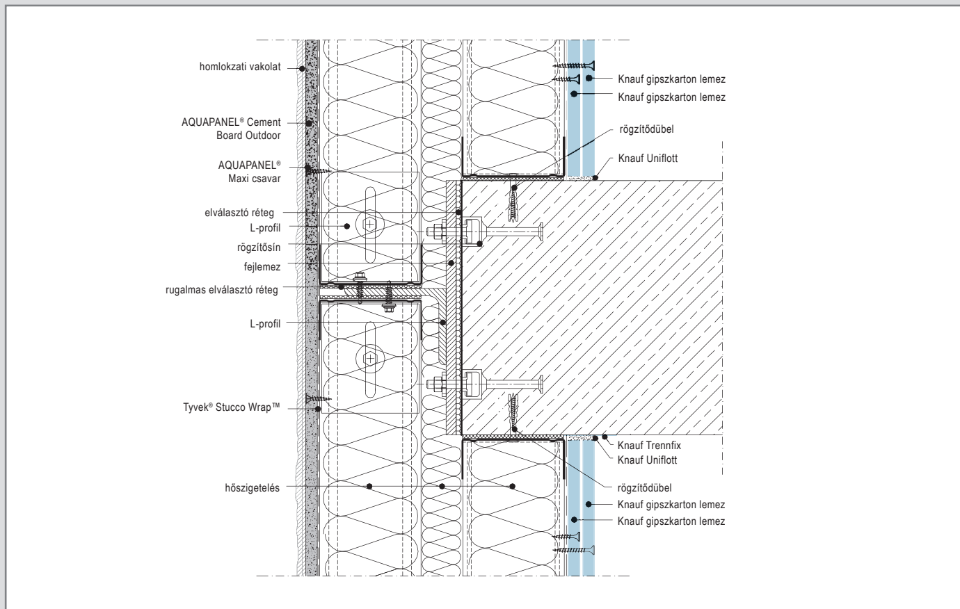
W388E-VM1 Födémcsatlakozás L-profillal, fejlemezzel
