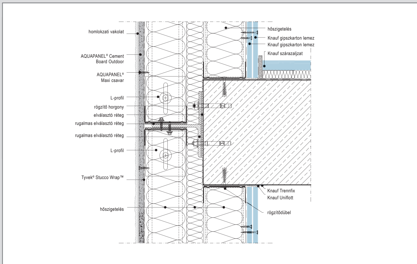
W388E-VM2 Födémcsatlakozás L-profillal közvetlen rögzítéssel
