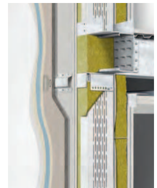
Kiszellőztetett homlokzat perforált profilú egyszeres vázzal
