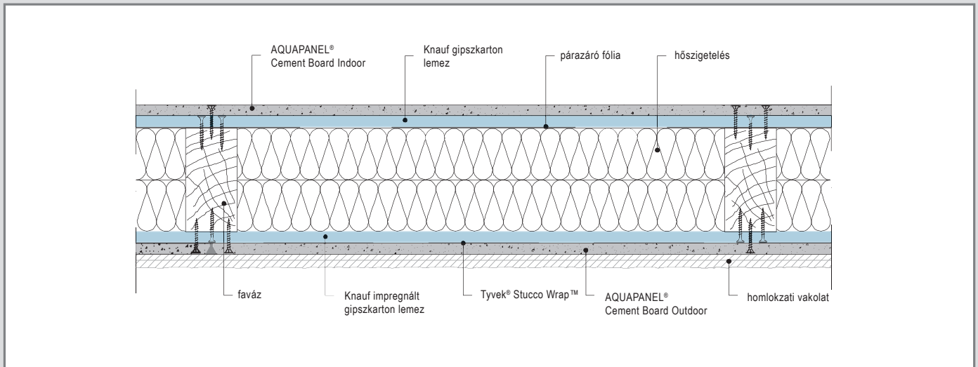
W572-H1 Alaprajzi kialakítás
