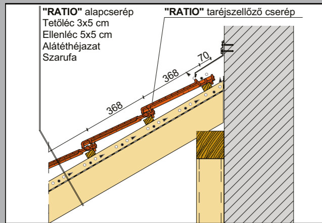
Falcsatlakozás
