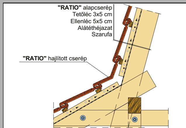
Hajlított cserép
